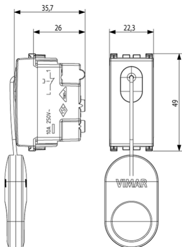
Vista ingombri
