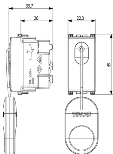
Vista ingombri
