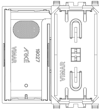
Vista posteriore
