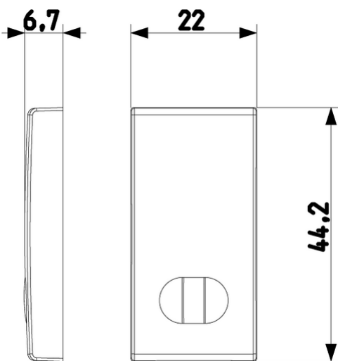
Vista ingombri
