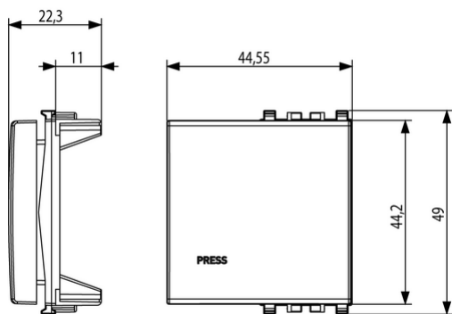
Vista ingombri
