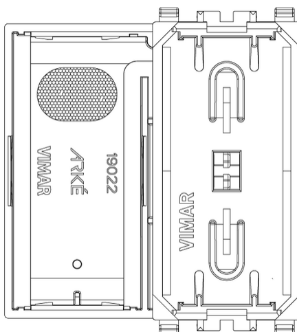
Vista posteriore
