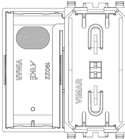
Vista posteriore
