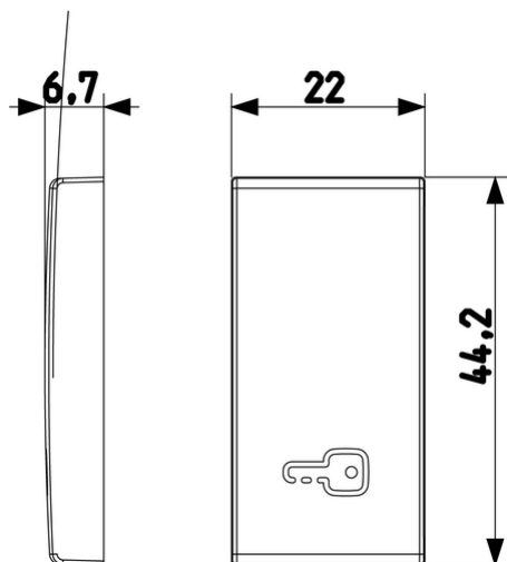
Vista ingombri
