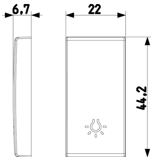
Vista ingombri
