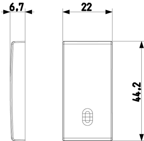
Vista ingombri
