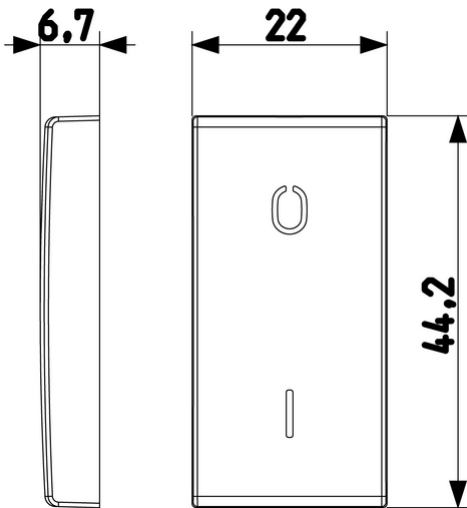
Vista ingombri
