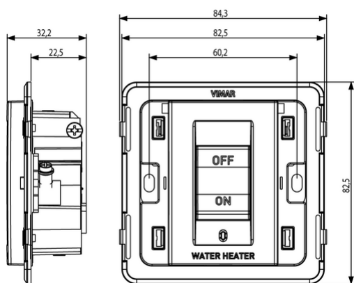
Vista ingombri
