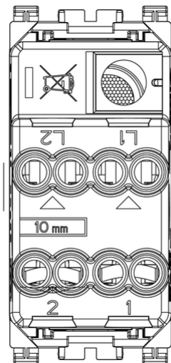
Vista posteriore
