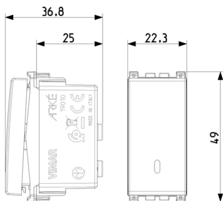
Vista ingombri
