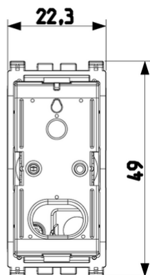
Vista ingombri
