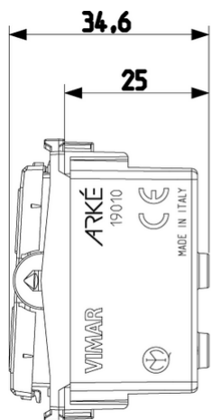
Vista ingombri
