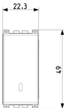
Vista ingombri
