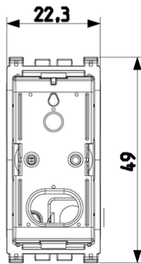
Vista ingombri
