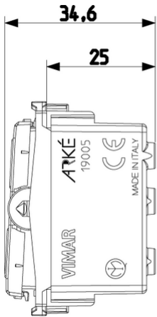
Vista ingombri
