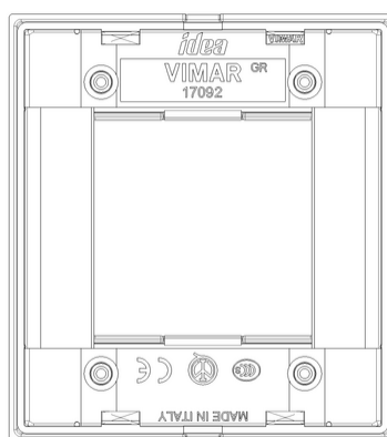
Vista posteriore
