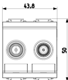
Vista ingombri
