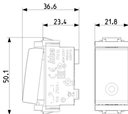
Vista ingombri
