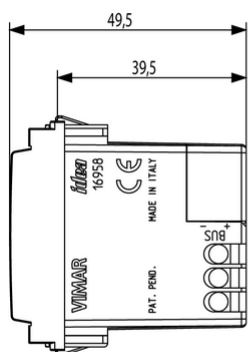
Vista ingombri
