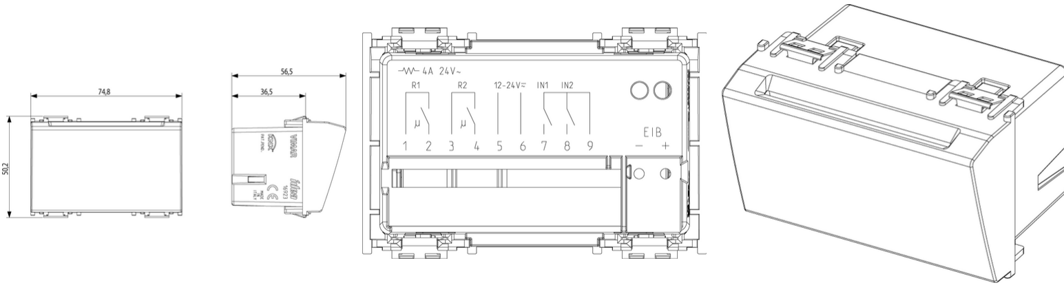
Vista ingombri
