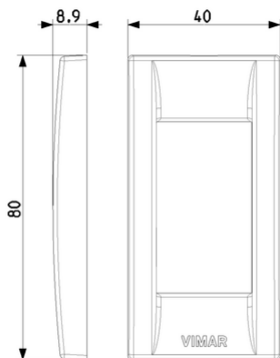
Vista ingombri
