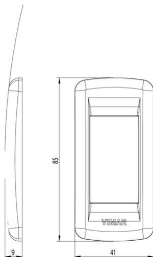
Vista ingombri
