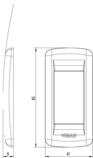
Vista ingombri
