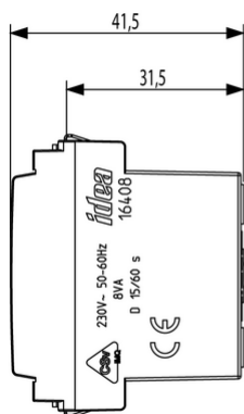
Vista ingombri
