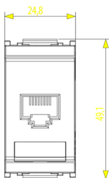
Vista ingombri
