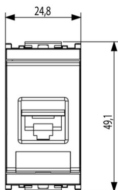
Vista ingombri
