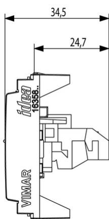
Vista ingombri
