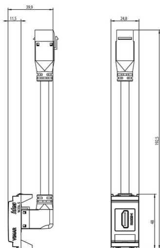
Vista ingombri
