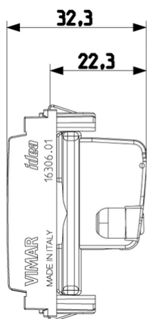
Vista ingombri
