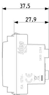
Vista ingombri
