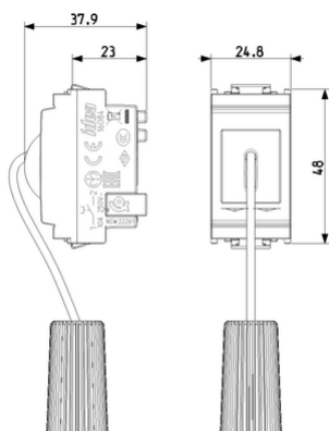
Vista ingombri
