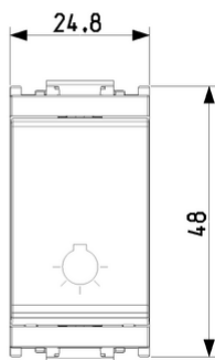
Vista ingombri
