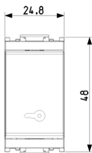
Vista ingombri
