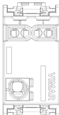
Vista posteriore
