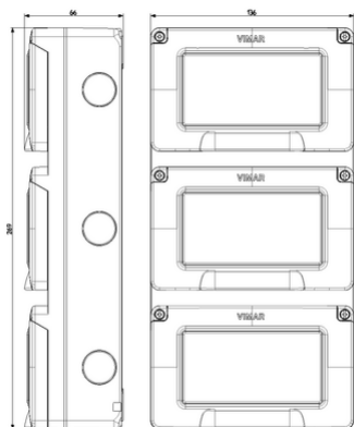
Vista ingombri
