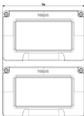
Vista ingombri
