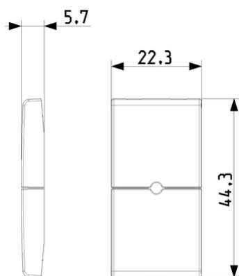
Vista ingombri
