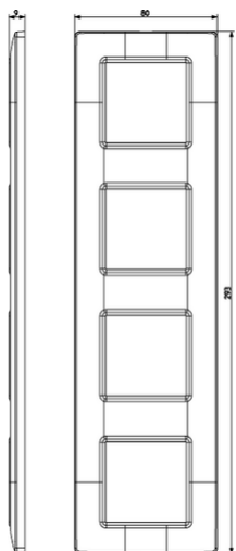
Vista ingombri
