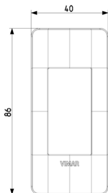
Vista ingombri
