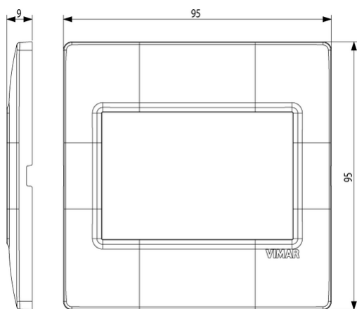
Vista ingombri
