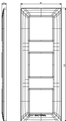
Vista ingombri
