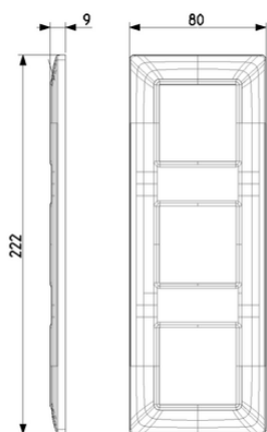
Vista ingombri
