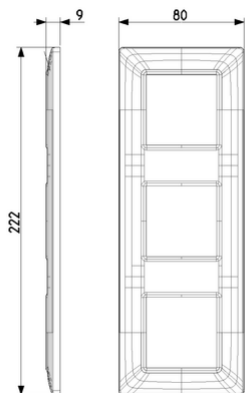
Vista ingombri
