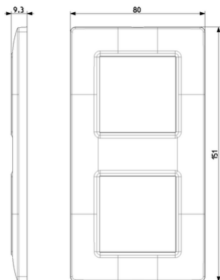
Vista ingombri
