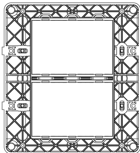
Vista posteriore
