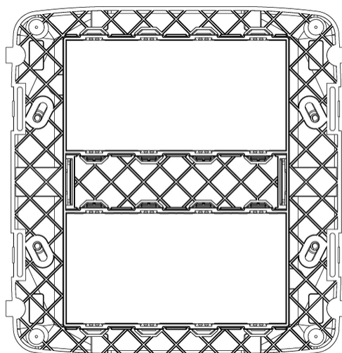
Vista posteriore
