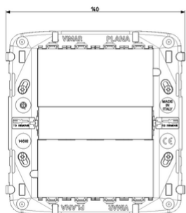
Vista ingombri
