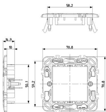
Vista ingombri
