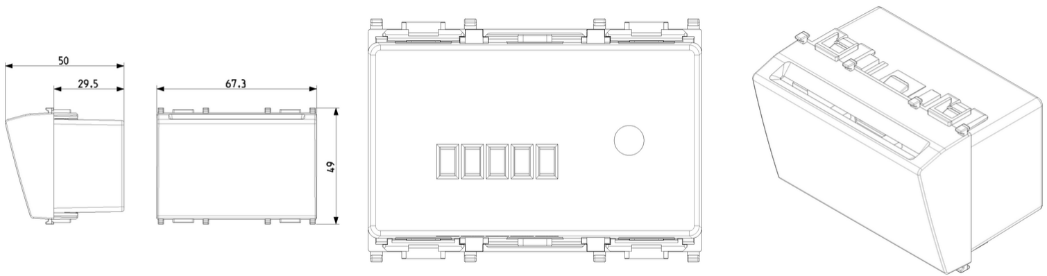
Vista ingombri
