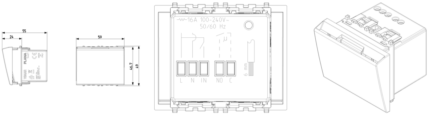
Vista ingombri
