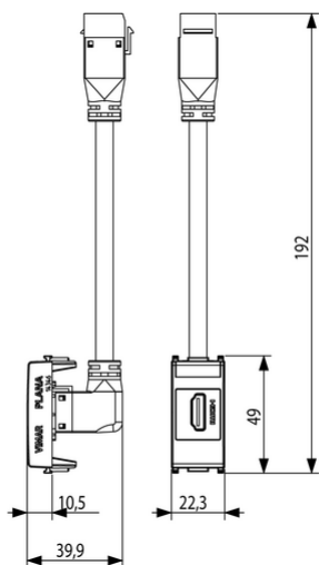
Vista ingombri
